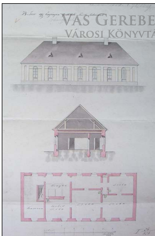
20. ábra: Várnagyi lakás, 1838.
