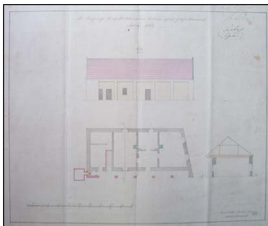
23. ábra: A mészároslakás újjáépítése, 1861.
