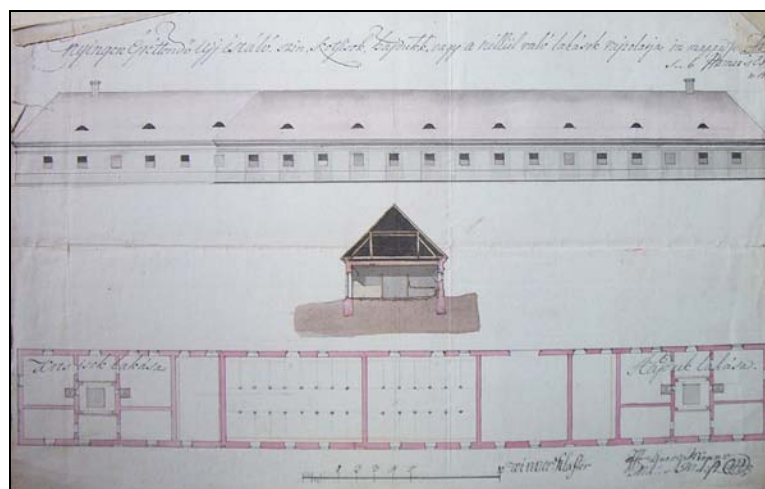
17. ábra: Az enyigyi új istálló rajza, 1849.
