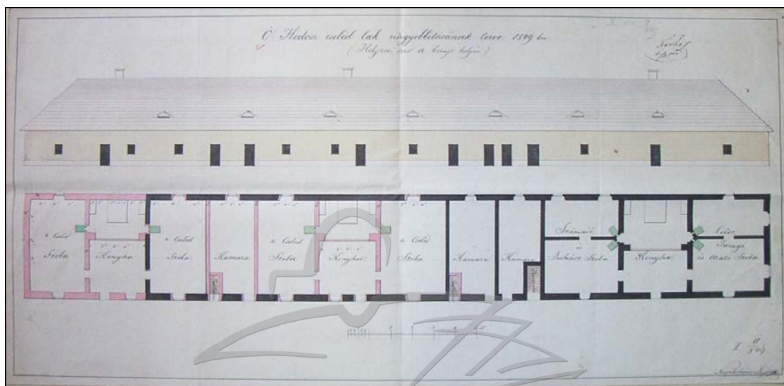
9. ábra: Az óhodosi cselédlakás megnagyobbításának terve, 1849
