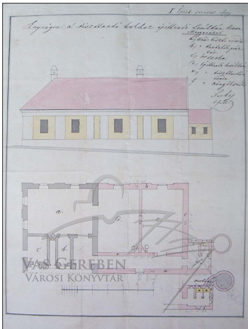
16. ábra: Tisztartói lakás levéltárral, 1834.
