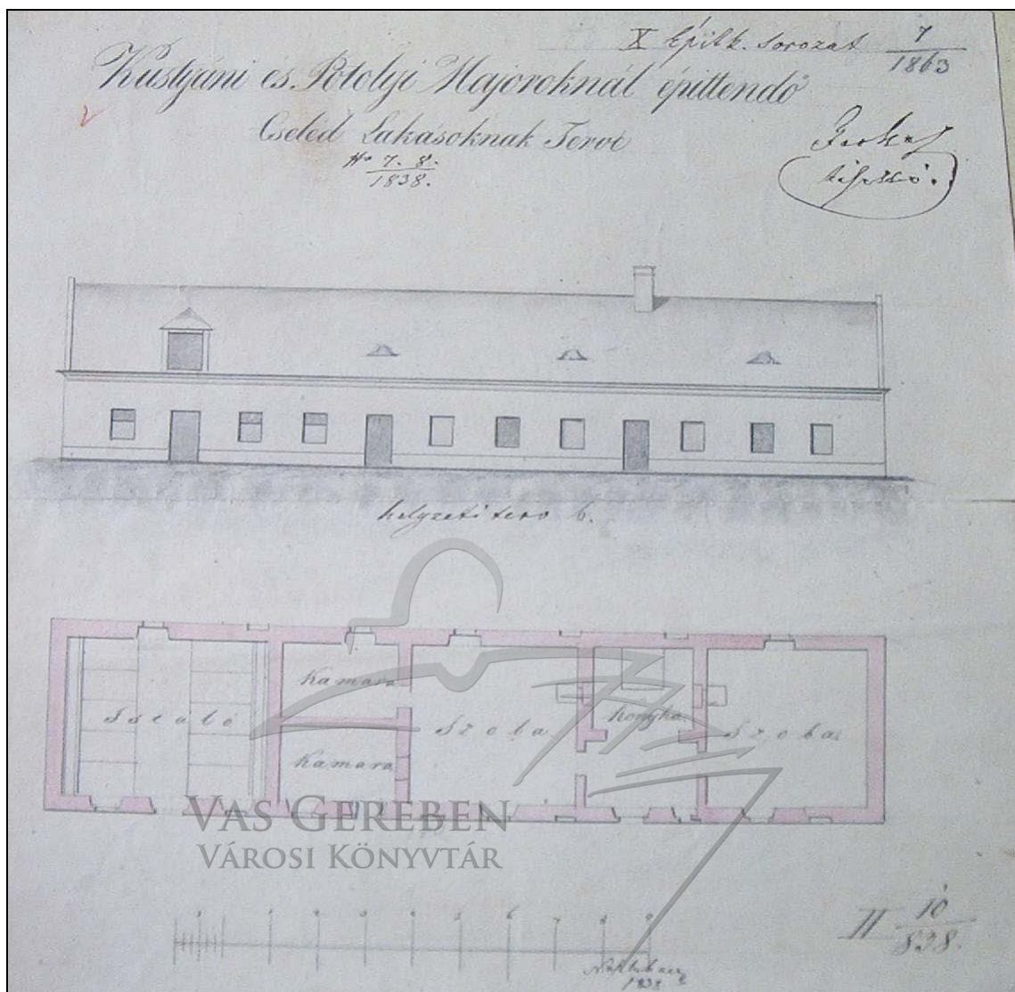
7. ábra: A kustyáni és potoli majorokban építendő cseléd lakás, 1838.
