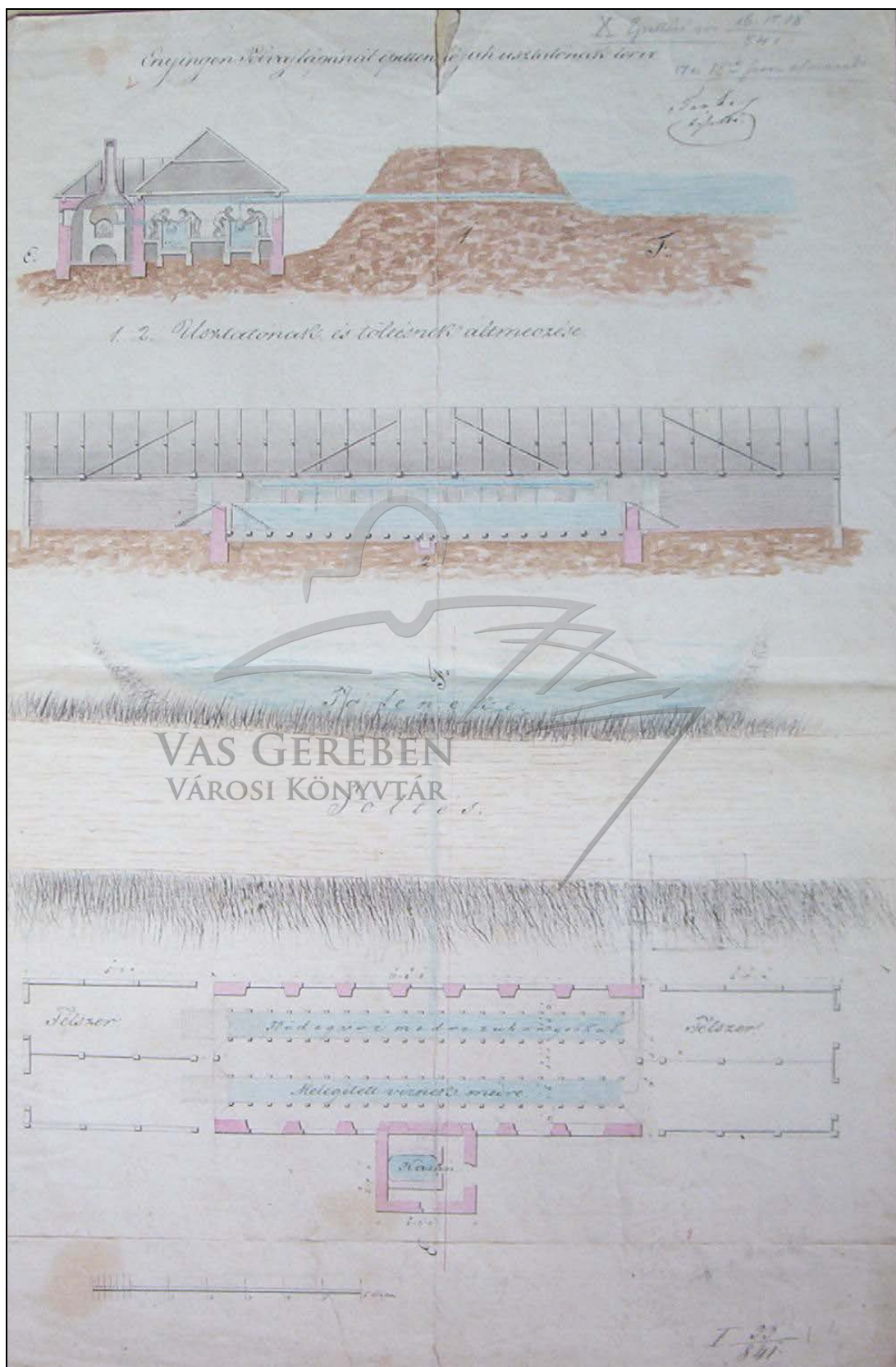
22. ábra: Az enyingi gyapjúmosó és úsztató, 1841-43.
