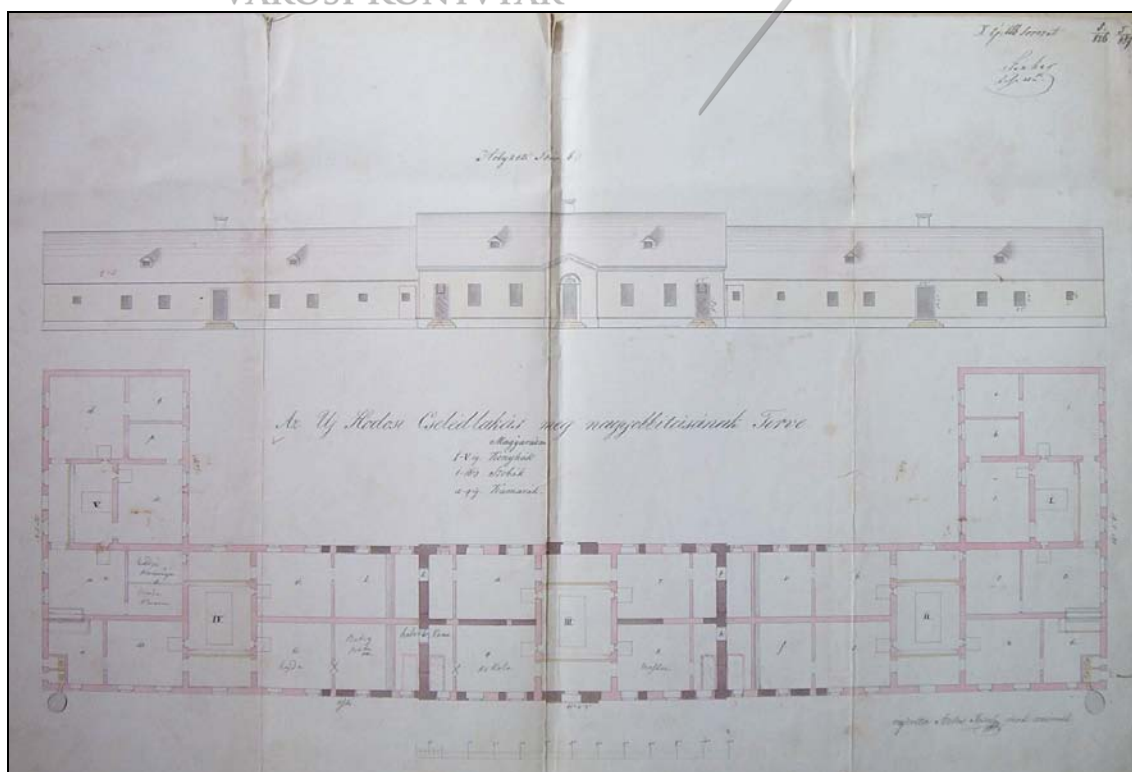
9. ábra: Az óhodosi cselédlakás megnagyobbításának terve, 1849
