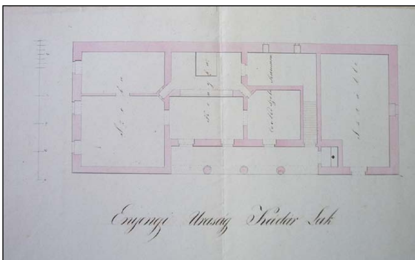
15 ábra: Az enyingi kádárlak
